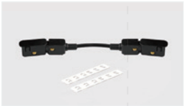
I-形供电连接器 (嵌入式) 型号: TLS-M265 尺寸: L70×W11.5×H2.1mm(拼接条) L78×W19×H17mm(供电包) 应用款型: TLS-MR2X0A TLS-MR2X0B TLS-MR2X0C
